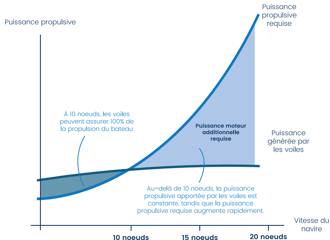
Vitesse et puissance propulsive générée grâce au vent
