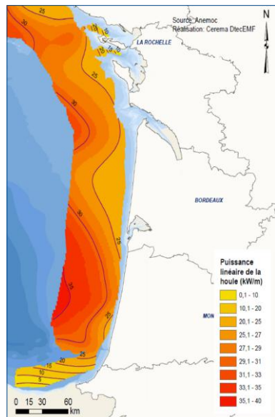
← Ressource pour les projets houlo-moteurs offshore : Puissance linéaire de la houle au large de la façade Sud-Atlantique (Source : données Anemoc - Cerema)
